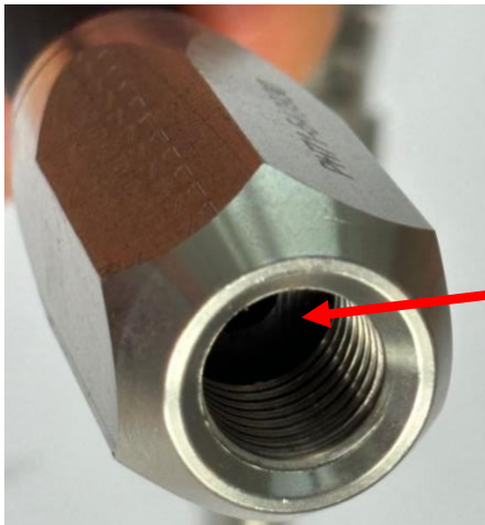
Abbildung 12 - Vormontierte Schraubfassung
