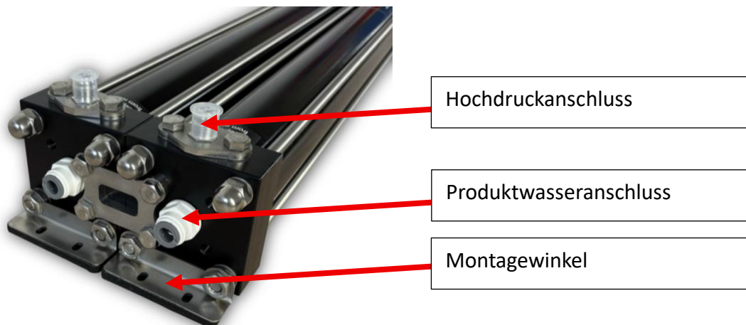
Abbildung 10 - Membraneinheit mit Anschlüssen für Seewasser und Produktwasser
