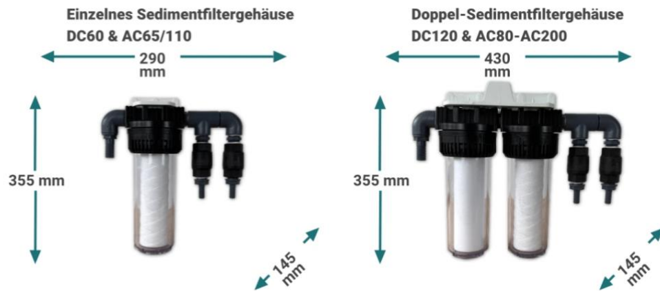
Abbildung 26 - Abmessungen Vorfiltergehäuse
