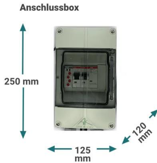
Abbildung 24 - Abmessungen Anschlussbox
