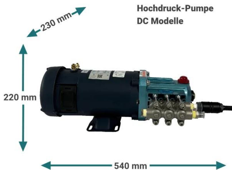
Abbildung 23 - Abmessungen Einheit Hochdruckpumpe
