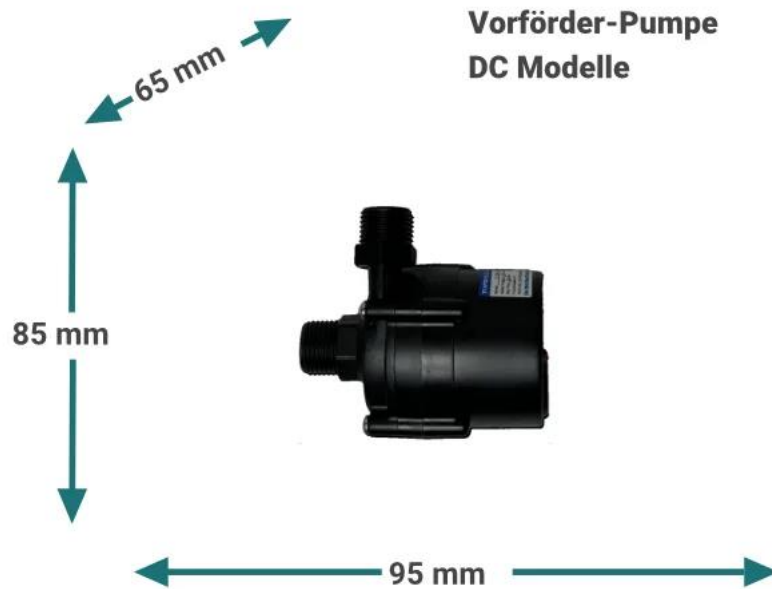
Abbildung 22 - Abmessungen Vorförderpumpe
