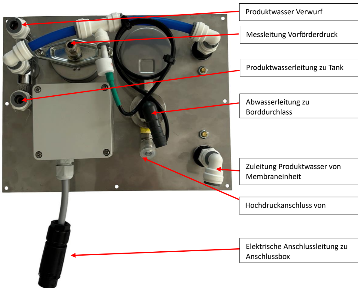
Abbildung 9 – Anschlüsse an Bedienteil
