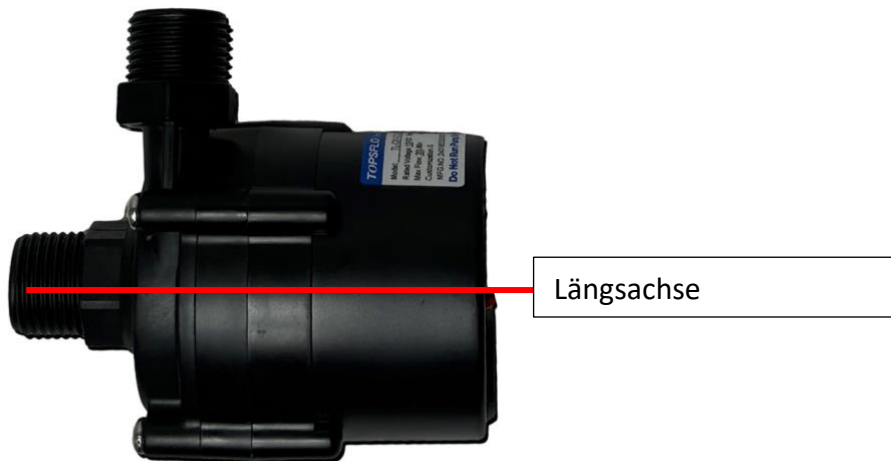
Abbildung 6 - Vorförderpumpe mit horizontal ausgerichteter Längsachse und Einlass, Auslass nach oben zeigend
