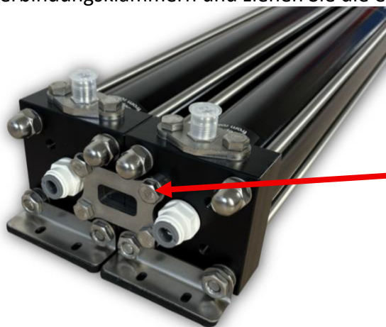
M8 Schrauben Verbindungsklammer
