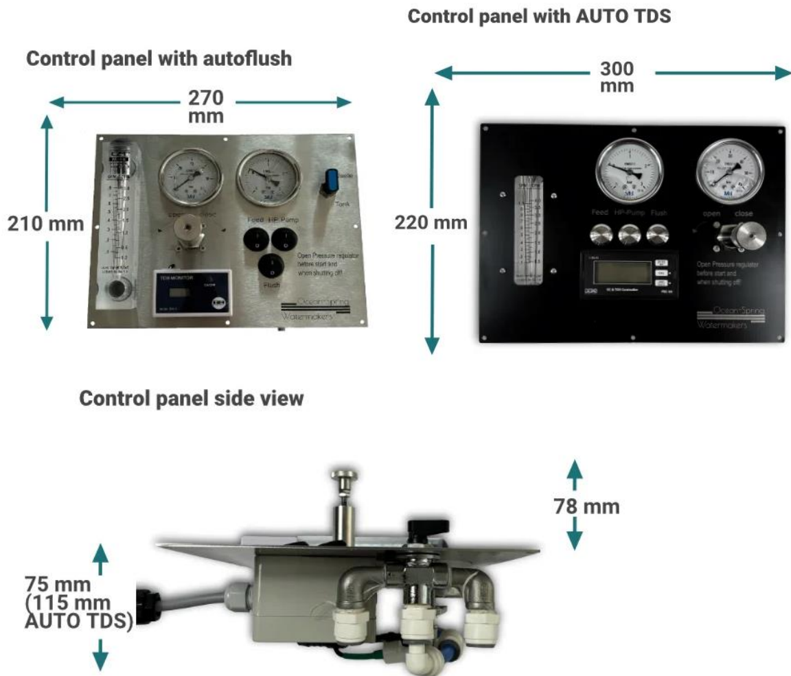
Abbildung 20 - Maße Bedienpanel
