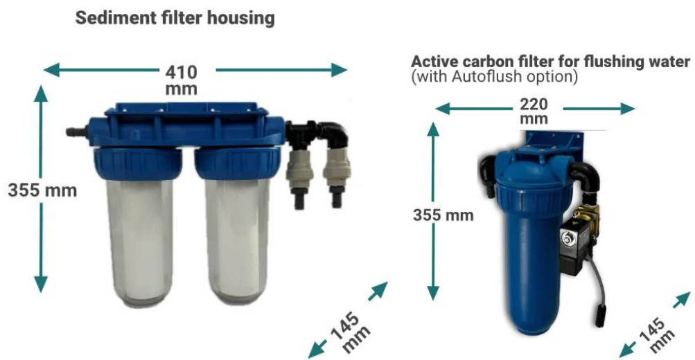
Abbildung 27 - Abmessungen Filtergehäuse
