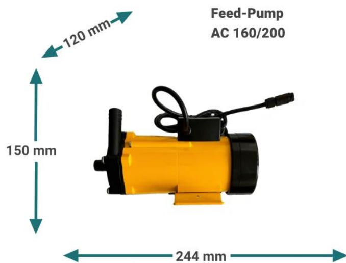
Abbildung 23 - Abmessungen Vorförderpumpe
