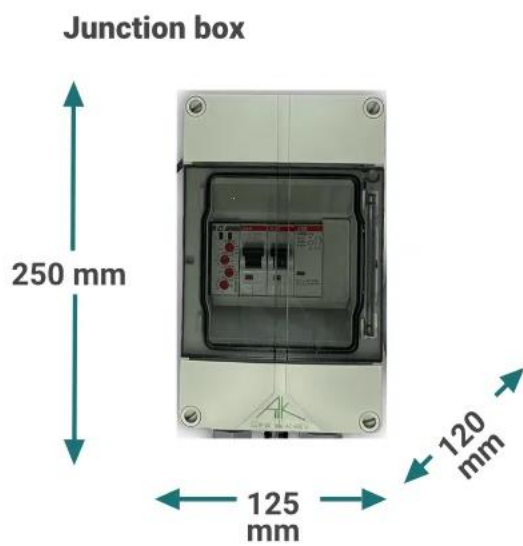
Abbildung 25 - Abmessungen Anschlussbox
