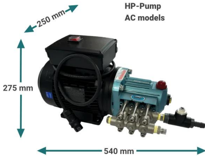
Abbildung 24 - Abmessungen Einheit Hochdruckpumpe
