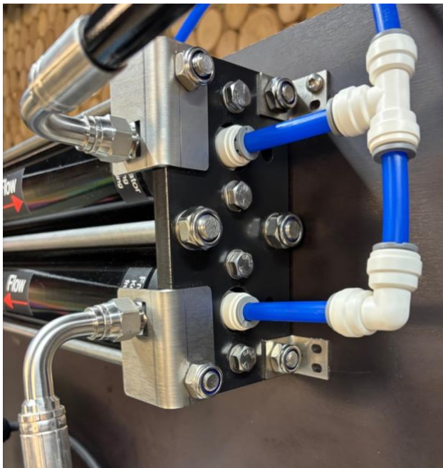
Abbildung 11 - Membraneinheit mit Anschlüssen für Seewasser und Produktwasser
