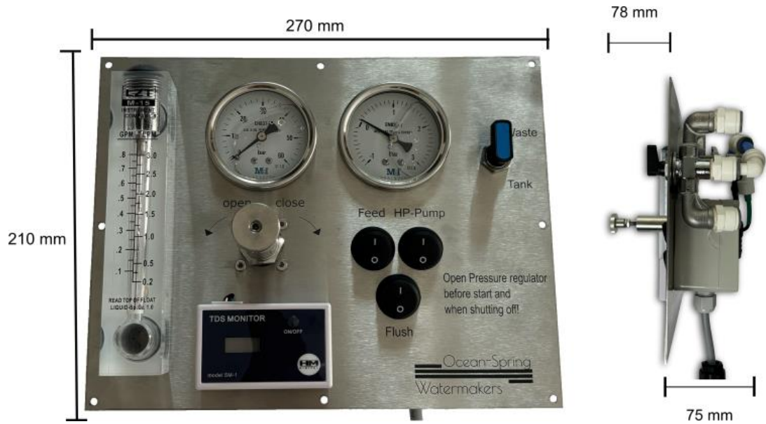
Abbildung 17 - Maße Bedienpanel
