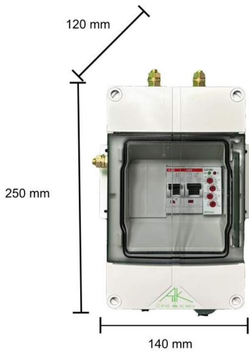
Abbildung 23 - Abmessungen Anschlussbox
