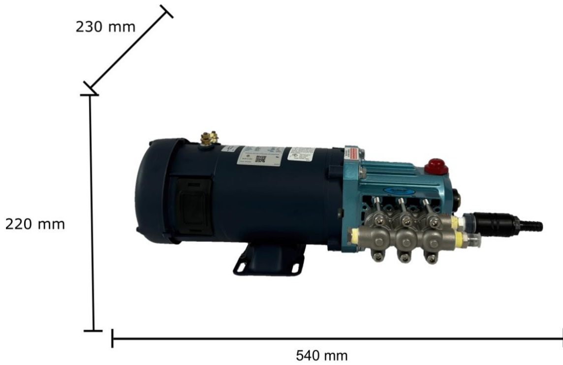
Abbildung 22 - Abmessungen Einheit Hochdruckpumpe
